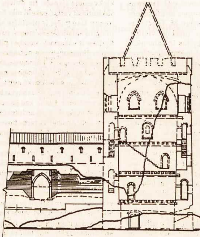
Medininkų Pilis. Šiaurinė siena iš kiemo pusės M 1 : 100
