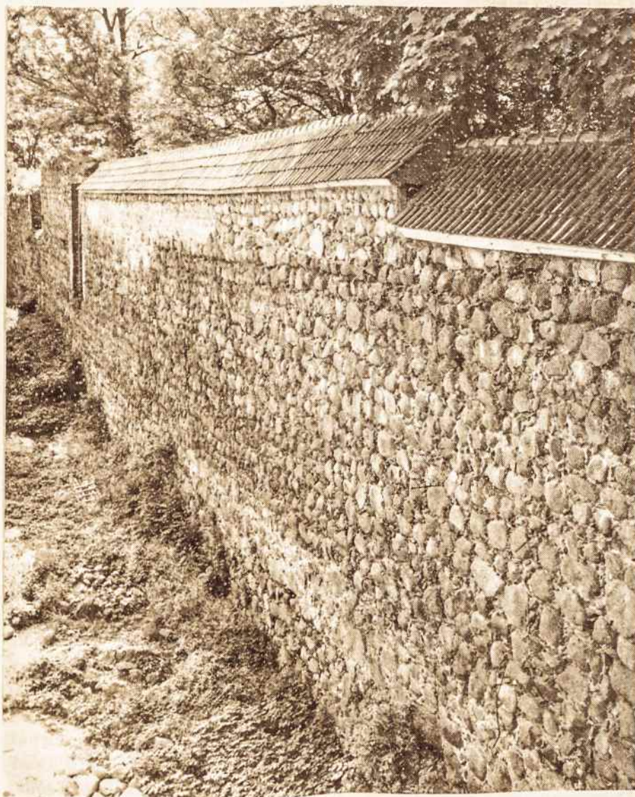
Restauruotos pietinės sienas fragmentas.
