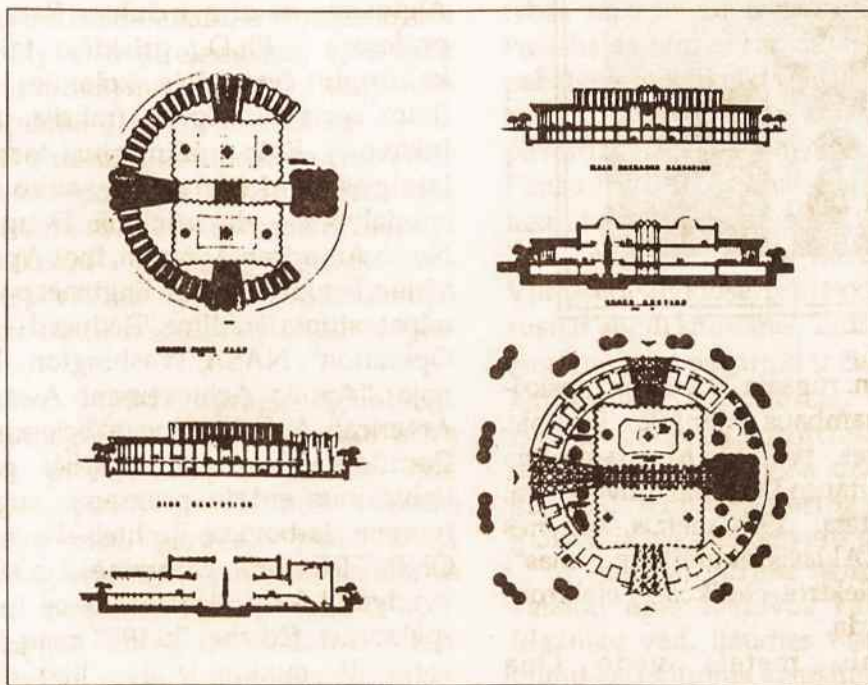
Konkursinis JAV pavilijono projektas New Yorko pasaulinėje parodoje. Konstrukcija išmontuojamų gelžbetoninių plokščių. Arch. Edm. Arbo projektas
