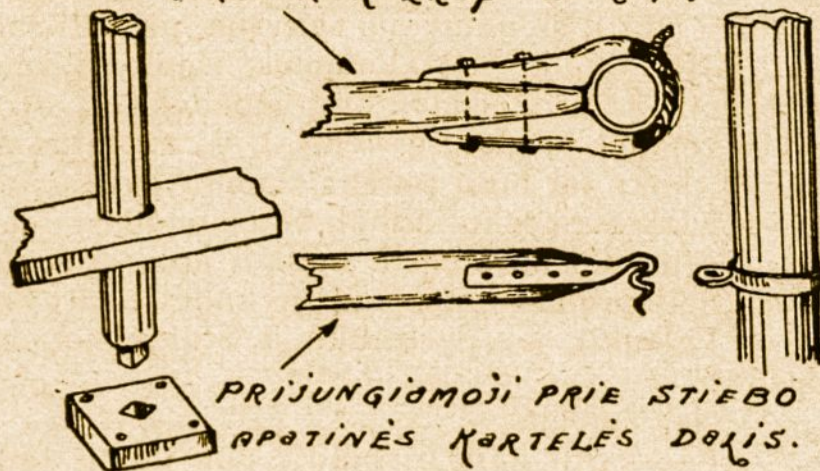
Brėž. 3. Sutvirtinimas burės kartelių su stiebu.
