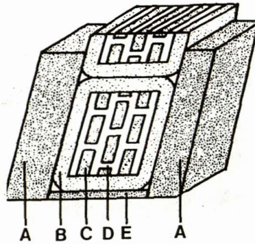
Chobham šarvo struktūra
