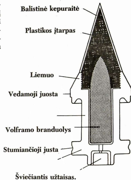
3A. Vokiečių sukonstruotas, vėliau sovietų kopijuotas prieššarvinis sviedinys.
