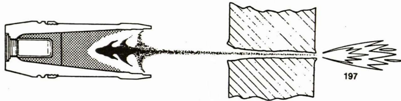
6A. Tuščiavidurio užtaiso veikimas: karštos sproginimo dujos pradegina šarvą.
