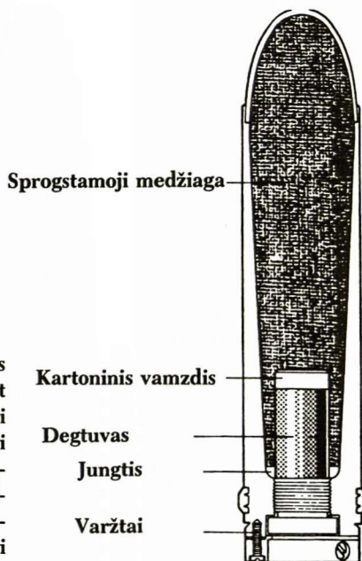
5. HESH – Prieššarvinė prisiplojanti granata
