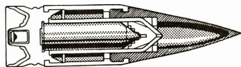
3B. Britų prieššarvinis sviedinys, kuriame lengvos dalys apsupta volframo branduolį.
