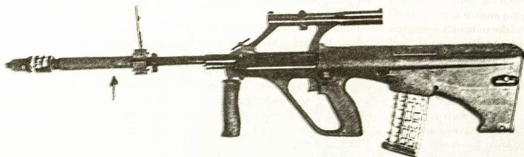
Austrių Steyr 5,56 mm AUG. Strėle pažymėta uždėta šaut. granata.
