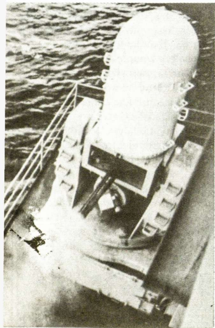
Labai efektingas 20 m m, MK 15, šešiavamzdis pabūklas
