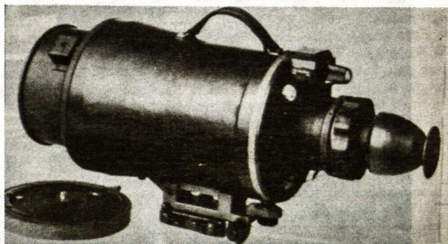
Prieštankinės artilerijos naktiniai taikytuvai, tikslūs iki 1400 metrų. Kairėje AN/TAS-4A prieštankinei vairuojamai raketai, dešinėje SS59 tipo taikytuvai
