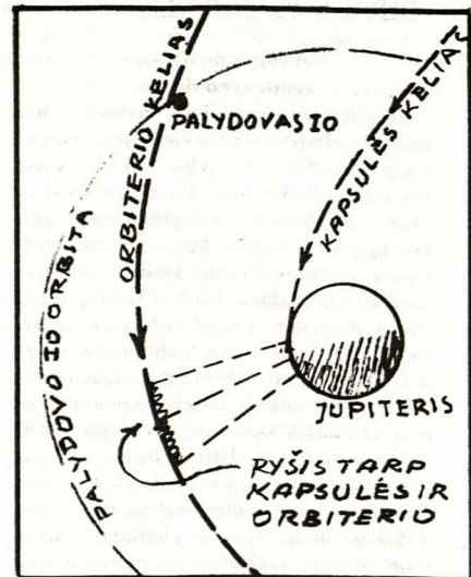
"Galileo" erdvėlaivio, orbiterio ir kapsulės keliai prie Jupiterio
