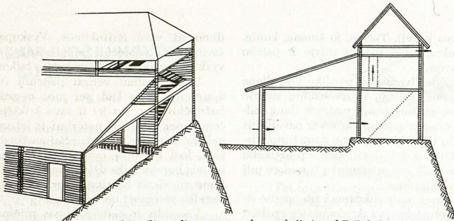
Jersikos pilies pylimo pastatų rekonstrukcija (pagal F. Balodį)
