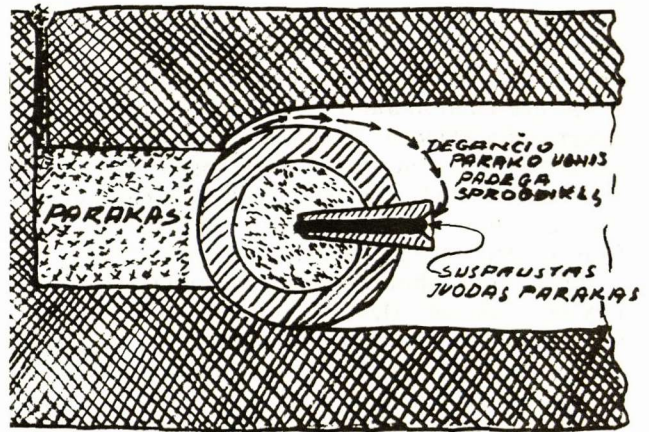
Patrankos skersinis pjūvis
