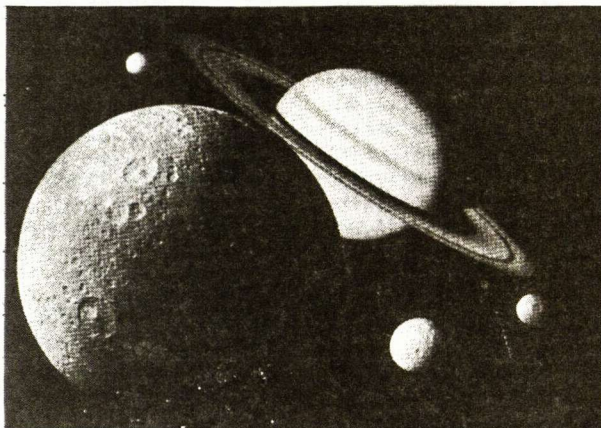
Saturnas su dalimi jo palydovų. Priekyje mėnulis Dione, dešinėje Tethys ir Mimas, kairėje viršuje — Enceladus ir Rhea. Tarp žiedų "Cassini" tarpas; ties planetos pusiauju, tamsus šešėlis.
