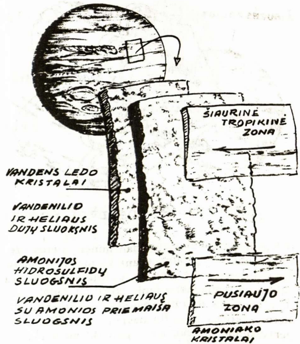
Jupiterio atmosferos klodai
