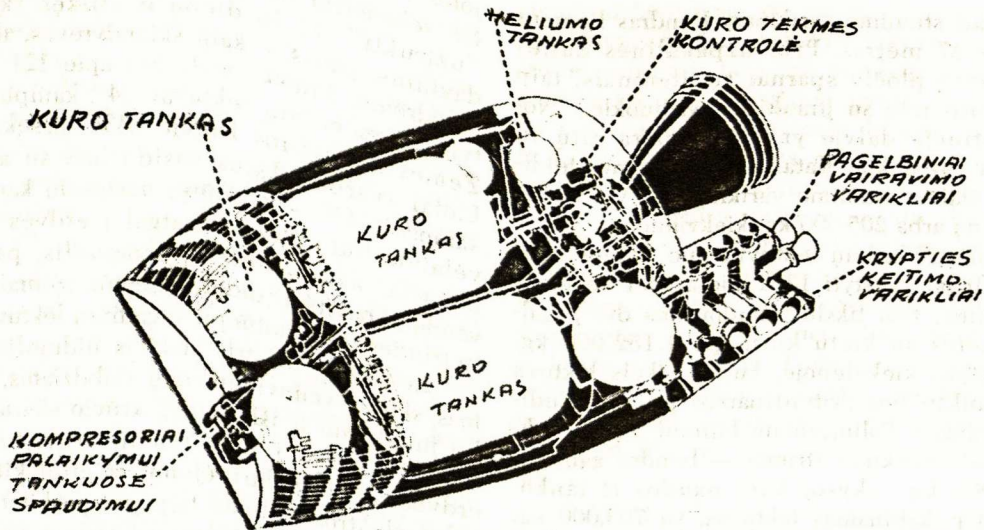
LEKTUVO UŽPAKALINIAI VARYMO IR VALDYMO VARIKLIAI
