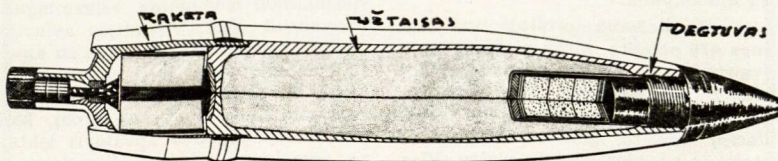
105 mm pabūklų sviedinio raketa veikia 1.8 sekundės, po 23 sekundžių palikus vamzdį.
