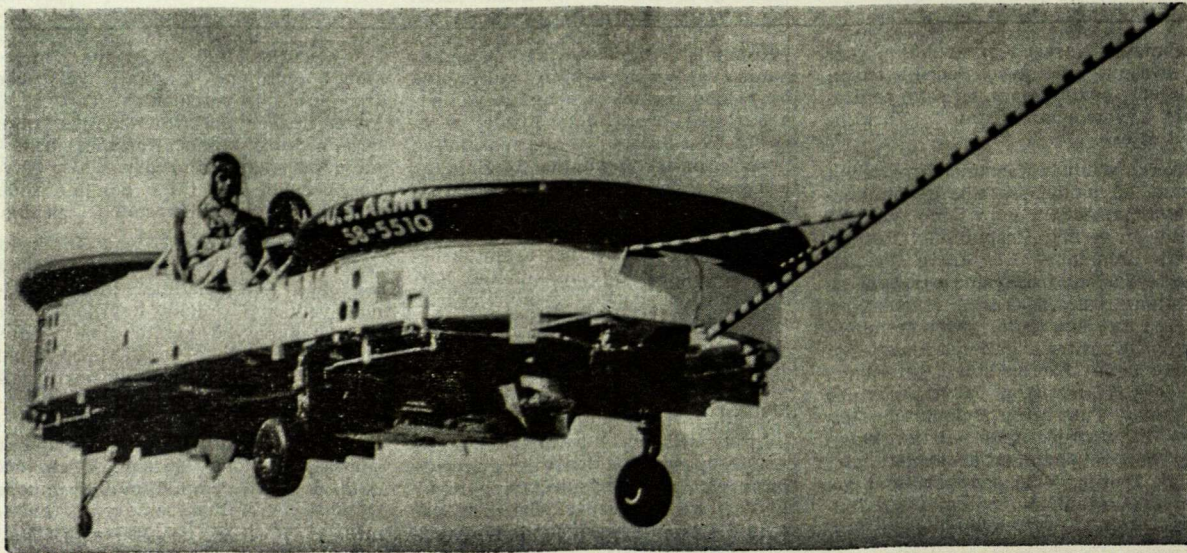
Orinis džypas, varomas turboprop motoro
