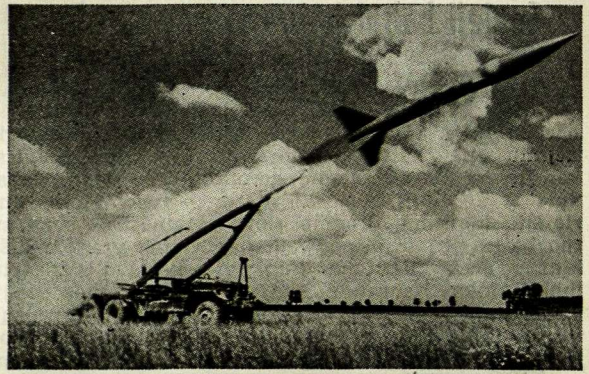
HONEST JOHN iššauinama nuo judraus stovo, manevrų metu Vokietijoje
