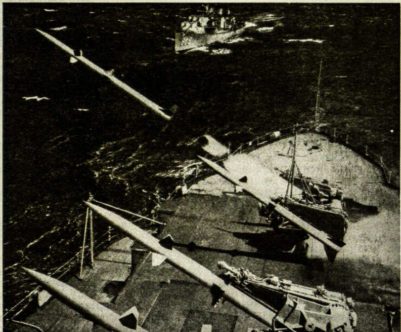
Vairuojama raketa TERIER , jūrų karinio laivyno išvystyta, vartojama ginkluoti naujausius JAV laivus.
