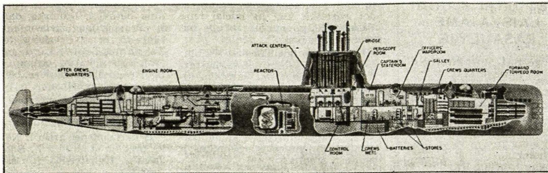
USS Nautilus, pirmasis povandeninis laivas, varomas atominė energija.
