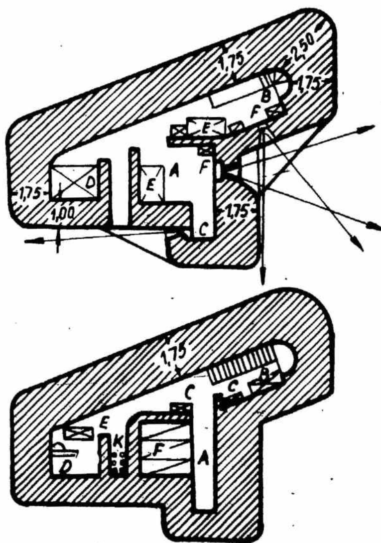
Br. 4. Dviejų aukštų kulkosvaidžių ugniavietė
