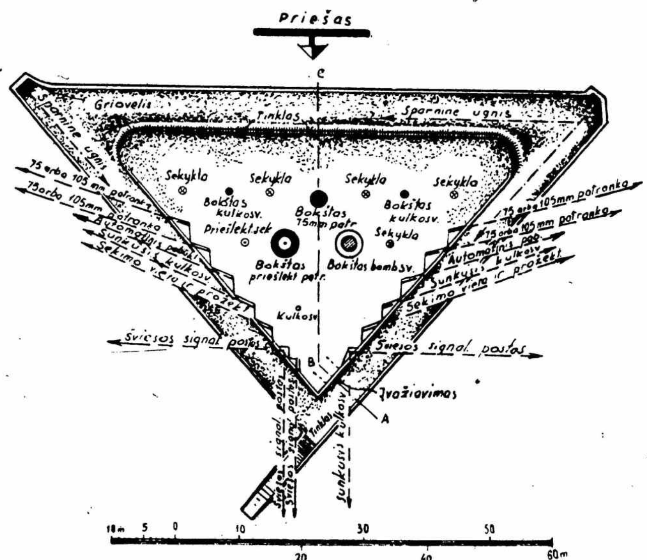
Br. 1. Tarpinis įtvirtinimas
