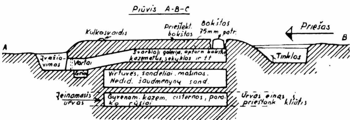
Br. 2. Tarpinio įtvirtinimo piūvis
