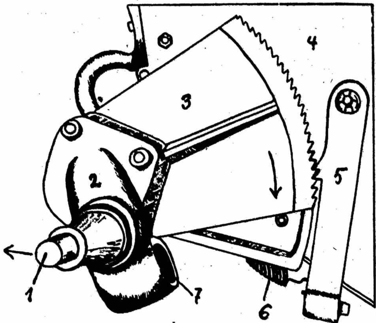
Br. 17. Vikšro įtempimo rato — įtempimo mechanizmas
