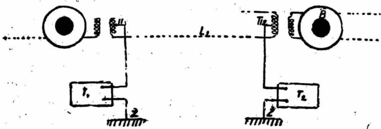
Br. 3. Simultaniam darbui tarp dviejų centrinių jungimo schema. A, B — telefono c-nės, L 1 , L 2 —telefono linijų laidai, Tr 1 , Tr 2 —transliatoriai, T 1 , T 2 —tolispaudžiai, Ž—žeminimas.
