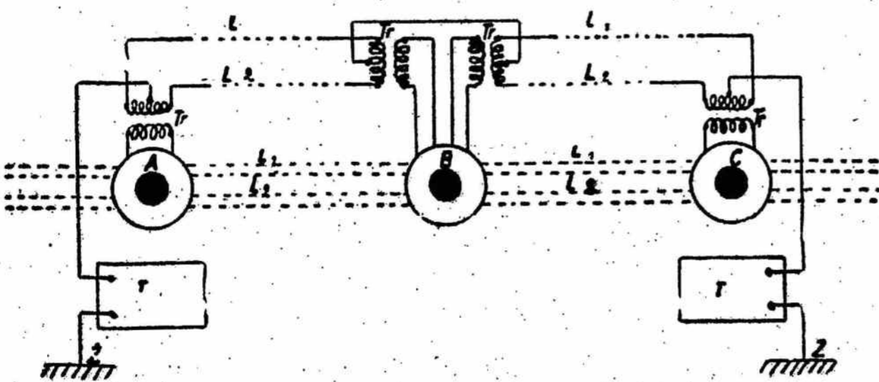
Br. 4. Simultaniam darbui tarp trijų ir daugiau telefono c-nių jungimo schema. Tr—transliatoriai, A, B ir C — telefono c-nės, L 1 , L 2 —telef. linijų laidai, T—tolispaudžiai, Ž—žemė
