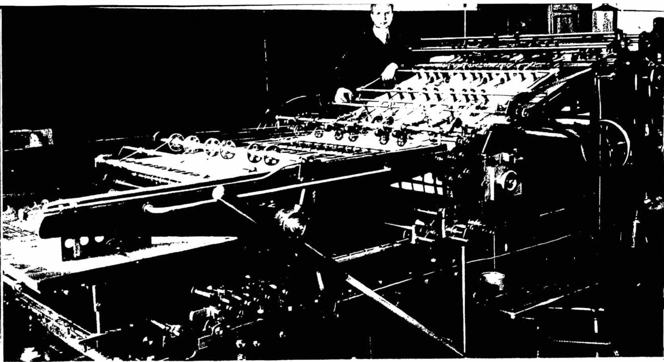
Didžioji mašina, iš karto spaudžianti 16 „Kario“ psl.
